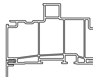
1/2" FLUSH FIN
